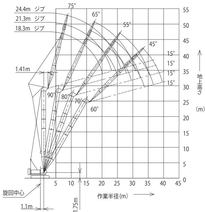
▶ ラッピングタワー定格総荷重表 (25.4tカウンタウエイト)
