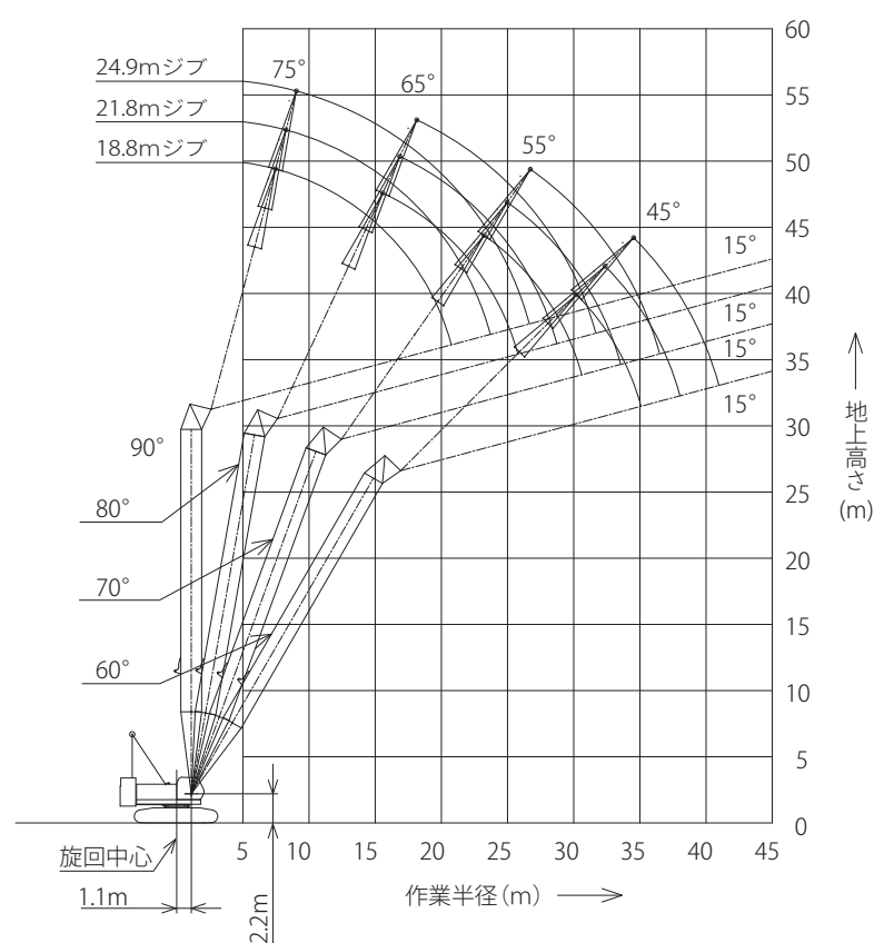
ラフティングタワー 定格総荷重表 (33.7t カウンタウエイト / カーボディウエイト装着) (単位：t)
