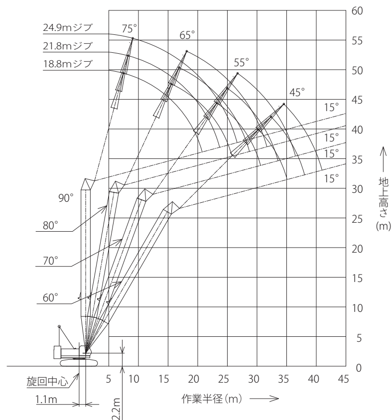
ラッフィングタワー 定 格 総 荷 重 表 (33.7t カ ウ ン タ ウ エ イ ト / カ ー ボ デ ィ ウ エ イ ト 装 着 ) (単 位 : t)
