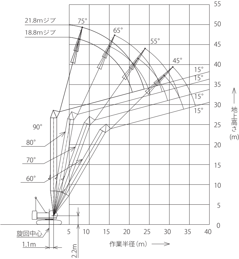
▶ ラッフィングタワー定格総荷重表 (33.7t カウンタウエイト / カーボディウエイト装着) (単位：t)
