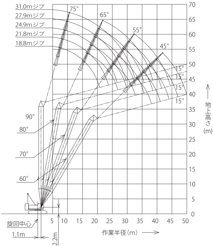
ラフティングターー定格総荷重表 (33.7t カウンタウエイト / カーボディウエイト装着) (単位：t)
