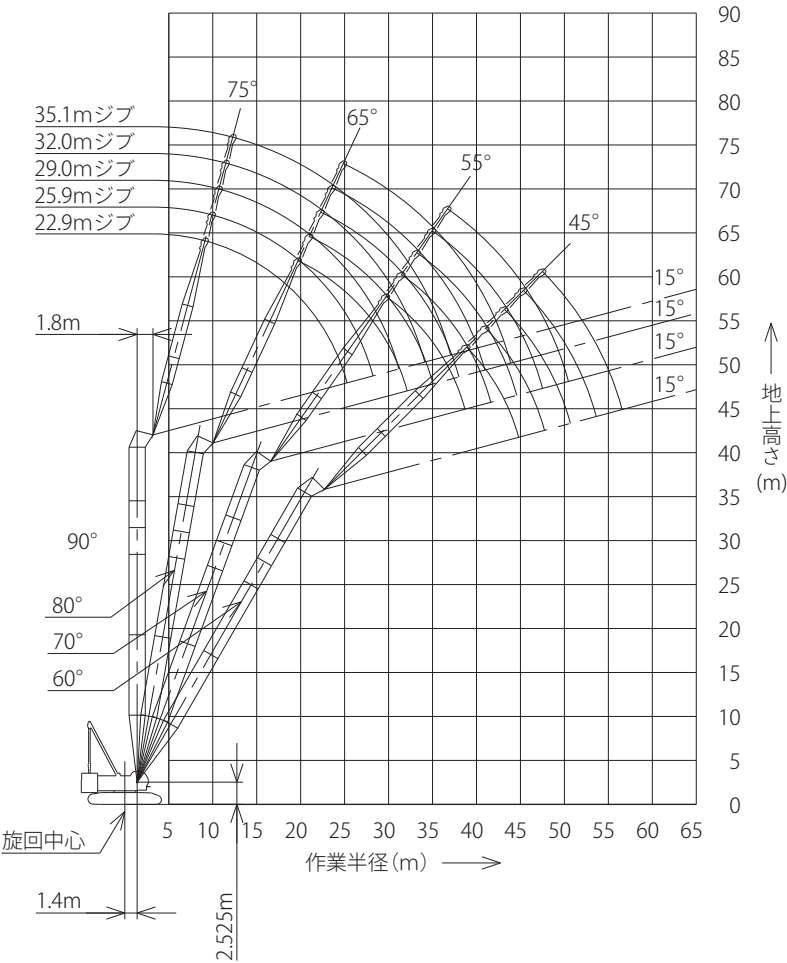
ラフティングタワー定格総荷重表
