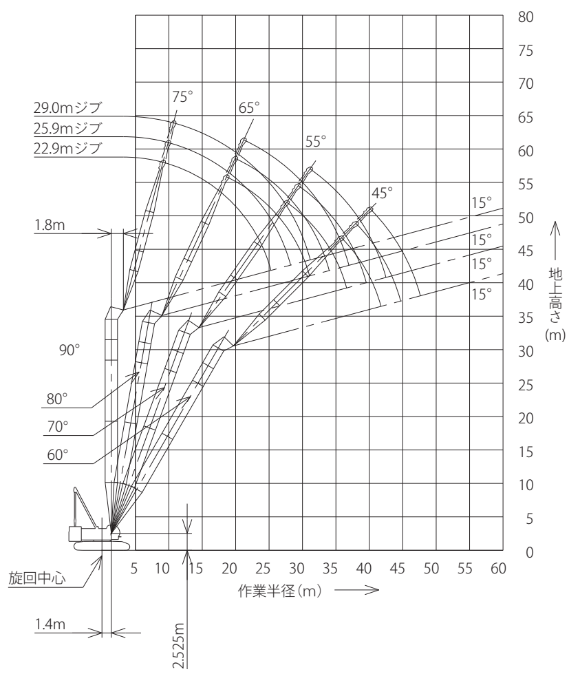
ラフティングタワー定格総荷重表
