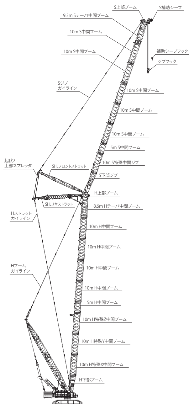
HL ラフティング 45+35m~95+85m
