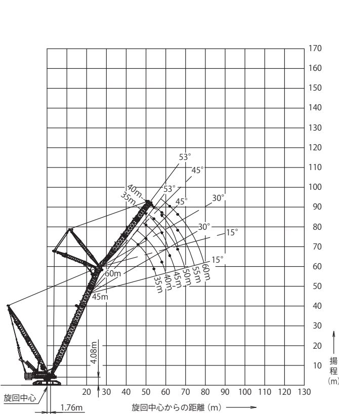
ラフティングジブ (ブーム角度 66°)
