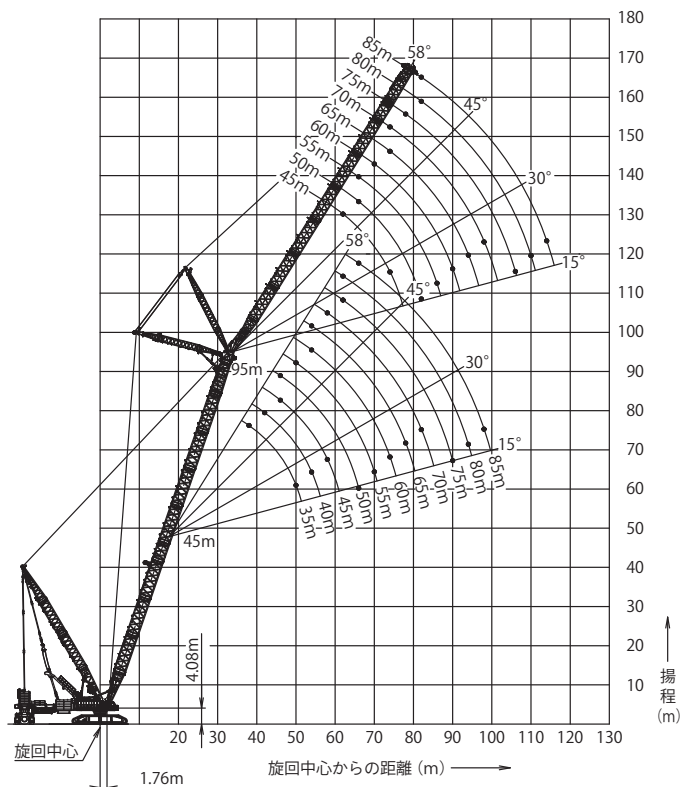
▶ ラッピングジブ （ブーム角度 71°）
