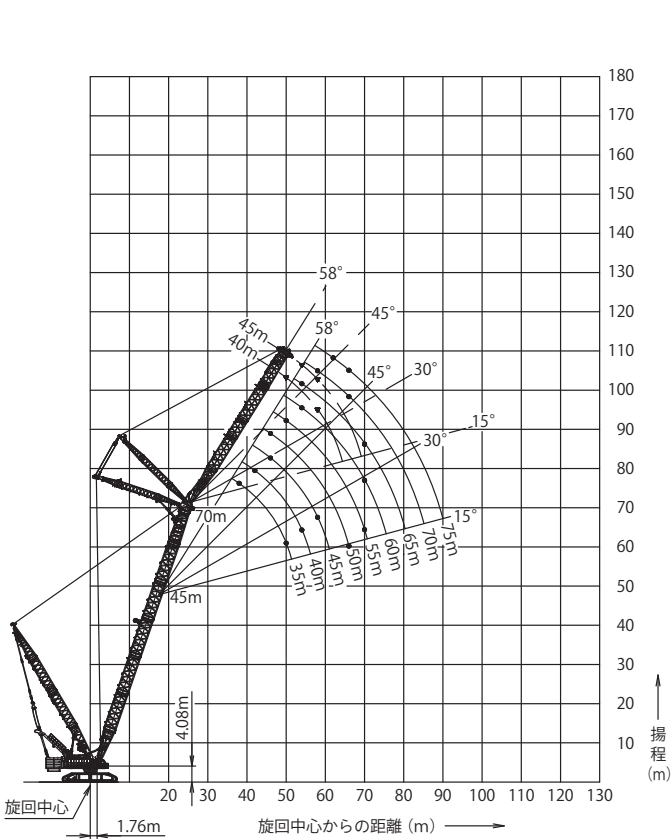
ラフティングジブ (ブーム角度 71°)
