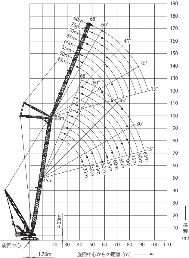
■ ラフティングジブ (ブーム角度 81°)
