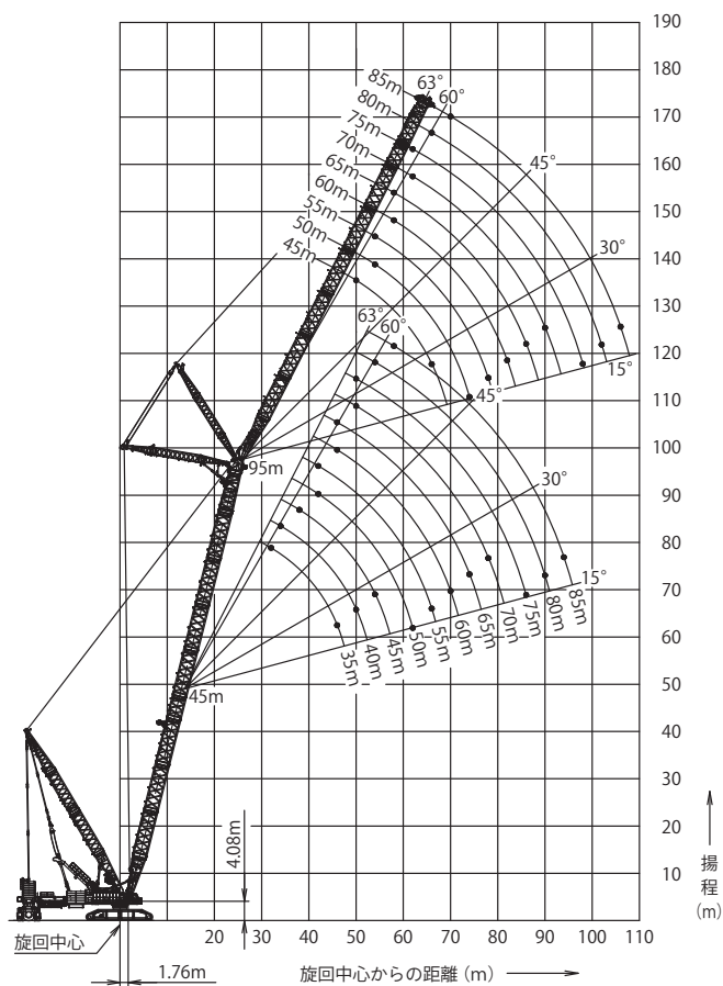
▶ ラッピングジブ （ブーム角度 76°）
