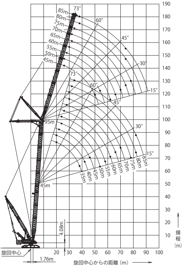
■ ラフティングジブ (ブーム角度 86°)
