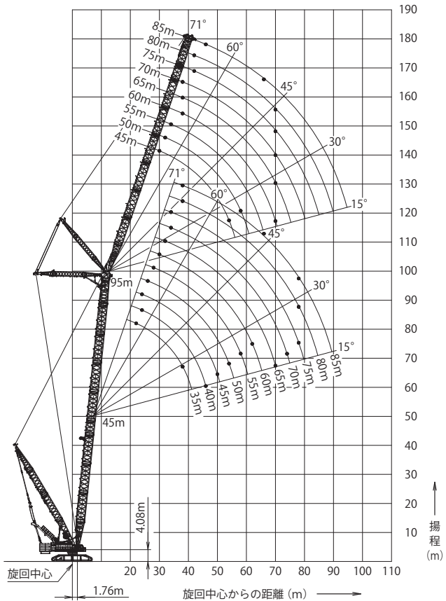
■ ラフティングジブ (ブーム角度 84°)
