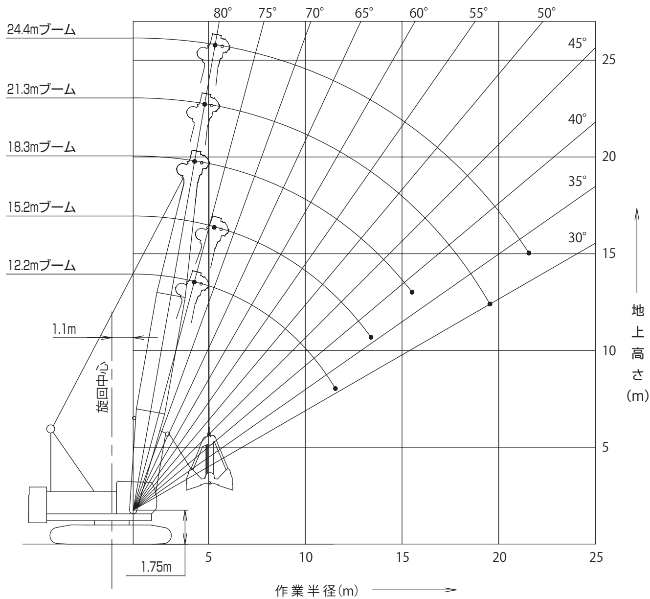
■ 作動範囲図
