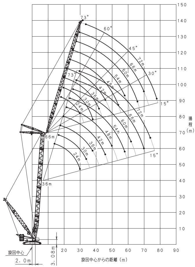
▣ ラフティングジブ（ブーム角度 86°）
