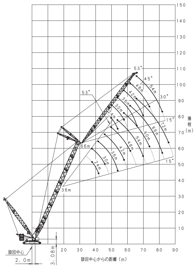
▣ ラフティングジブ（ブーム角度 66°）
