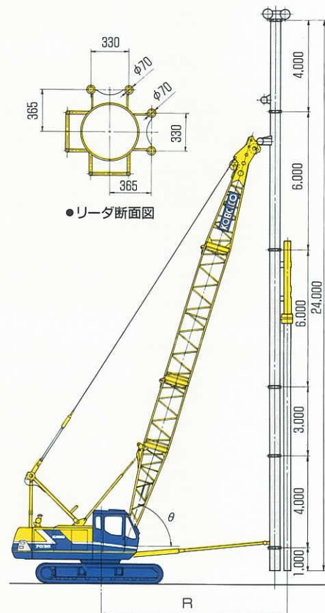
■2面パイルドライバ作業姿勢図(単位:mm)
