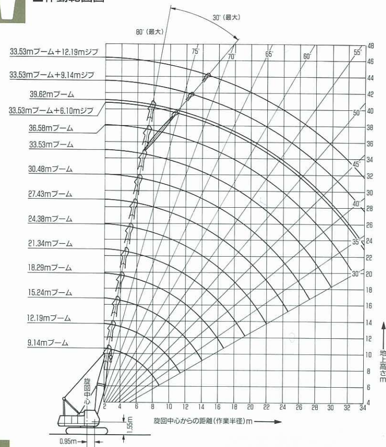
■作動範囲図
