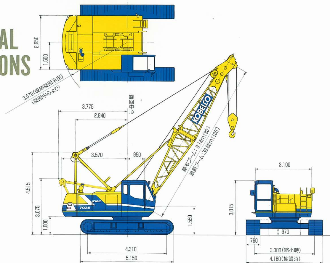
■全体図 (単位:mm)
