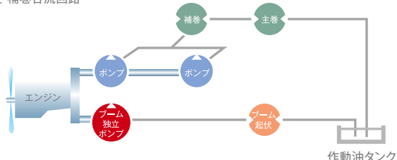
主・補巻合流回路
