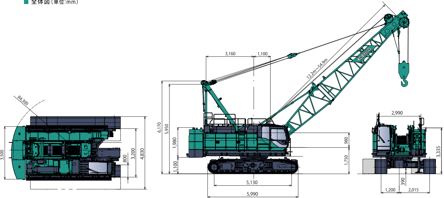
■ 全体図 (単位:mm)
