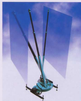
旋回角度の制限制御
