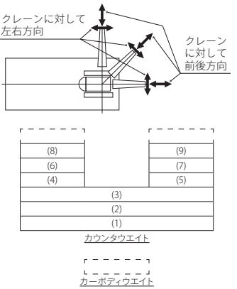
クラムシェル作業定格総荷重表 (53.1t カウンタウエイト/カーボディウエイトなし)
